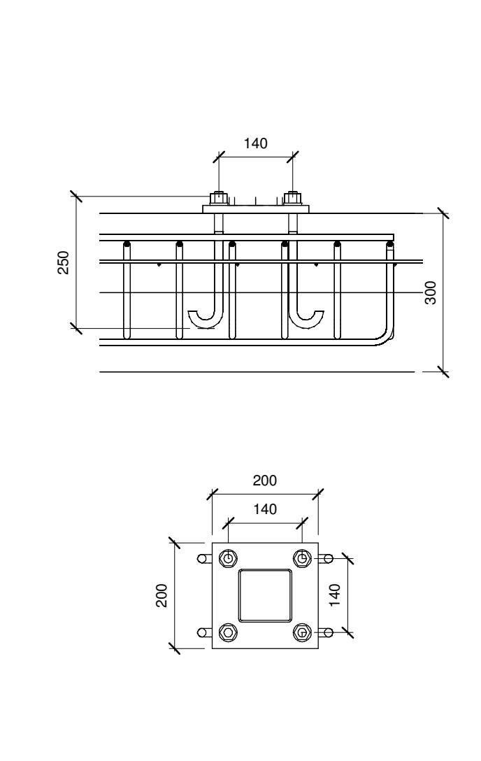
ΛΕΠΤΟΜΕΡΕΙΑ ΣΥΝΔΕΣΗΣ ΕΔΡΑΣΗΣ ΣΤΥΛΩΝ κλ.1:10 ΛΓΚΥΡΙΑ M16 / δ.8 - ΠΑΧΟΣ ΠΛΑΚΑΣ 15mm
