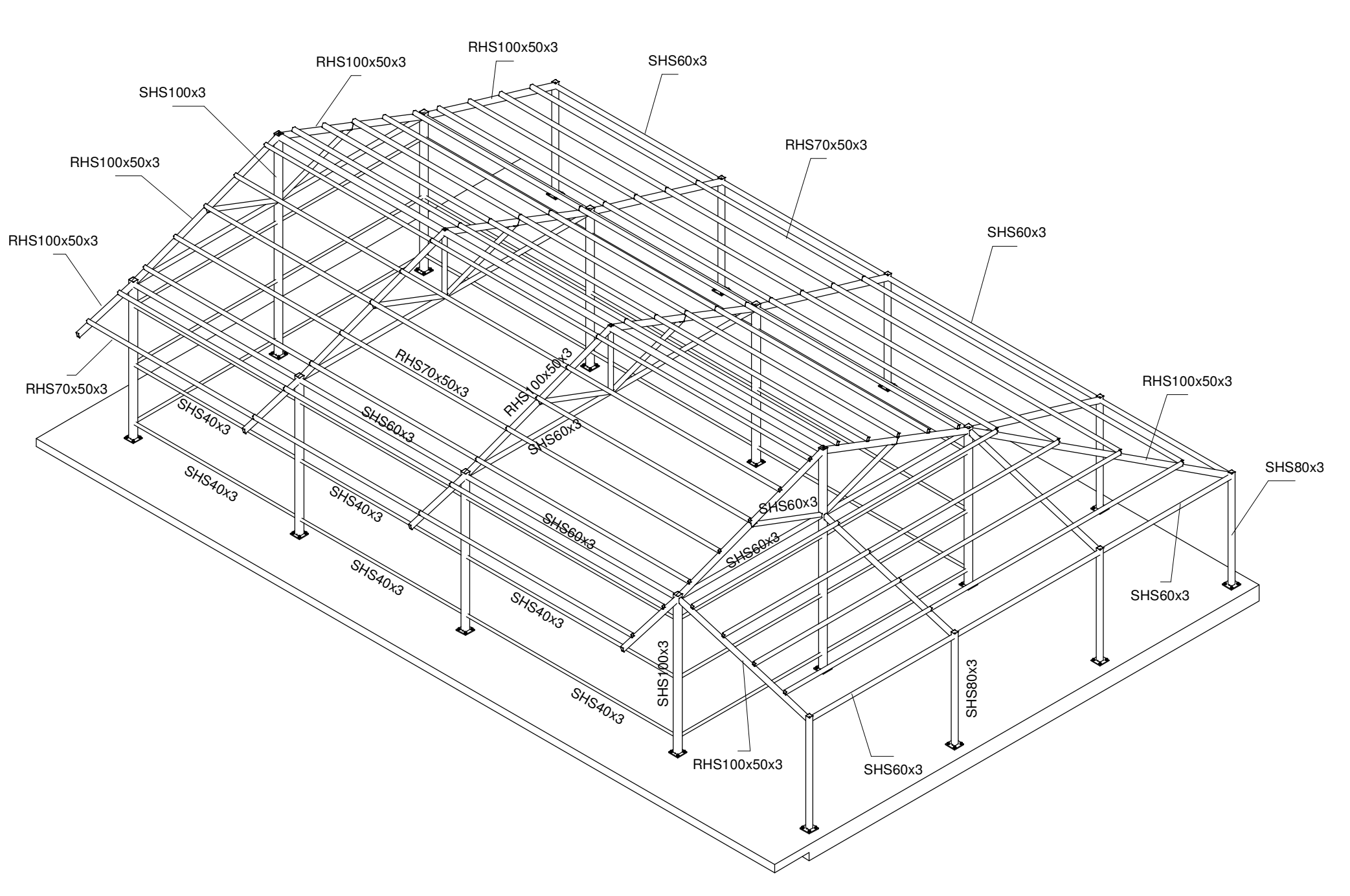
ΑΞΟΝΟΜΕΤΡΙΚΟ
