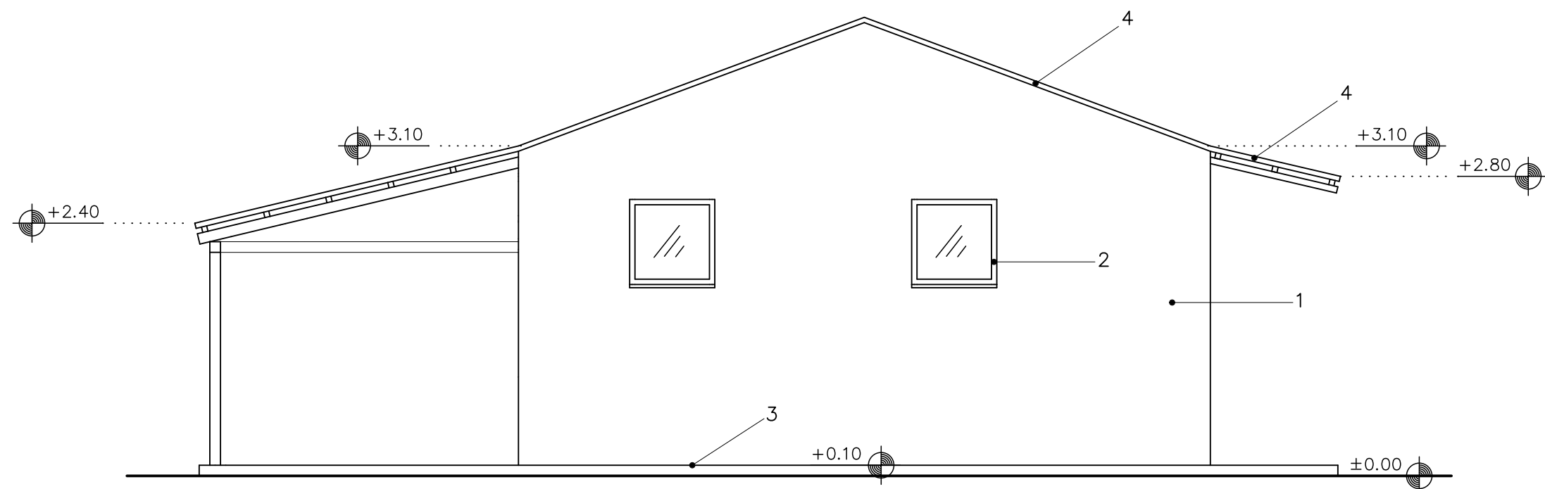
ΟΨΗ 2
