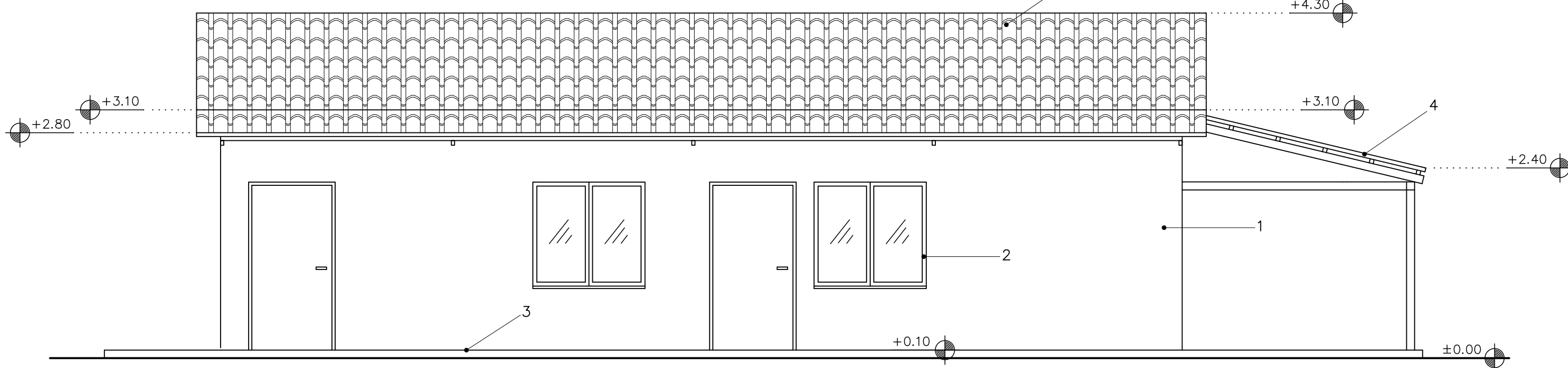
ΟΨΗ 1
