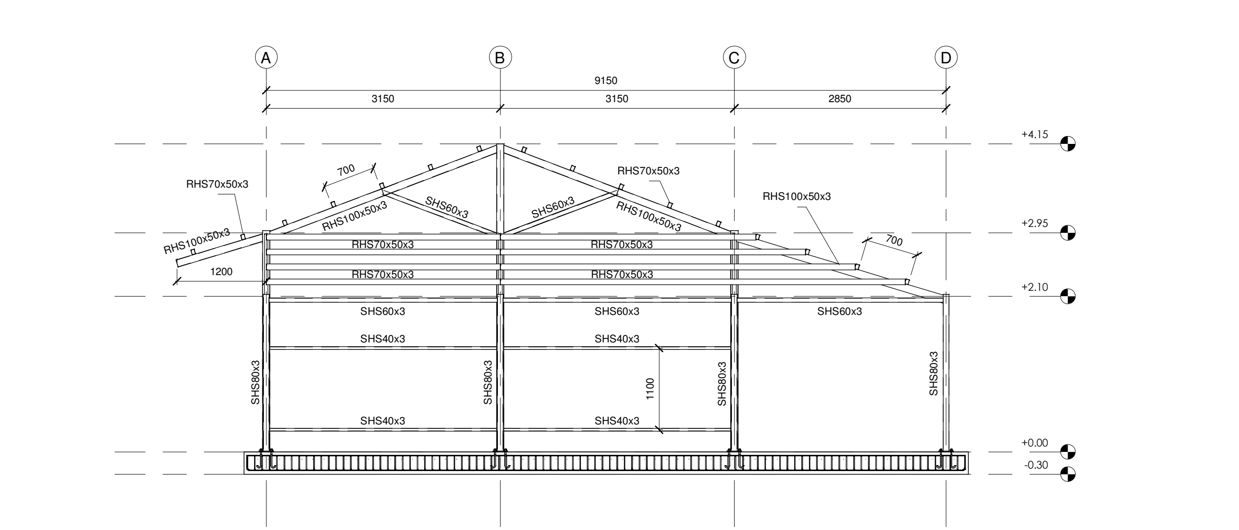
ΠΡΟΣΩΠΗ 1:50
