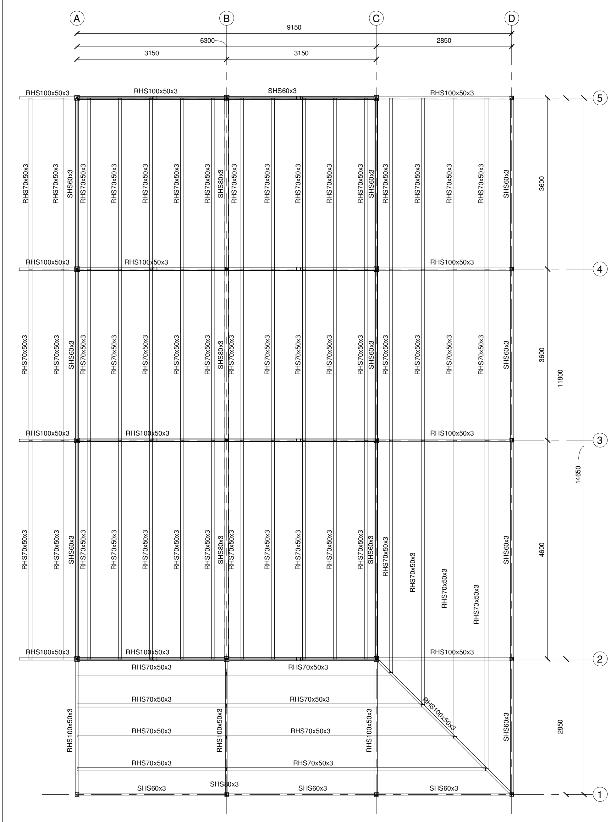
ΔΙΑΤΑΞΗ ΣΤΕΓΗΣ 1:50
