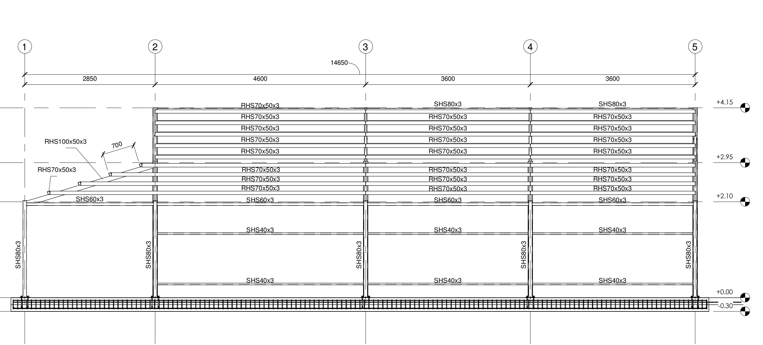
ΠΛΑΓΙΑ ΟΨΗ 1:50
